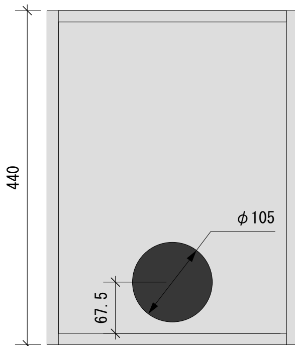
上面図
