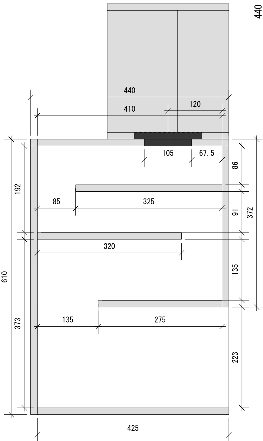
側面図
